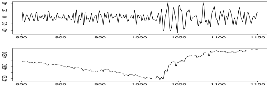
Fig. 4. A: Seismic signal. B: AIC value.
